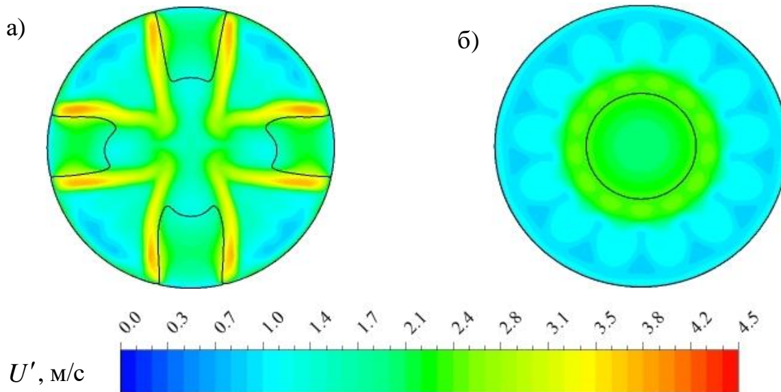
Рис. 12. Поля середньоквадратичних значень пульсацій швидкості U' в поперечному перерізі x = 0,275 м для паликового пристрою потужністю 110 кВт за наявності (а) і відсутності (б) турбулізаторів потоку.
