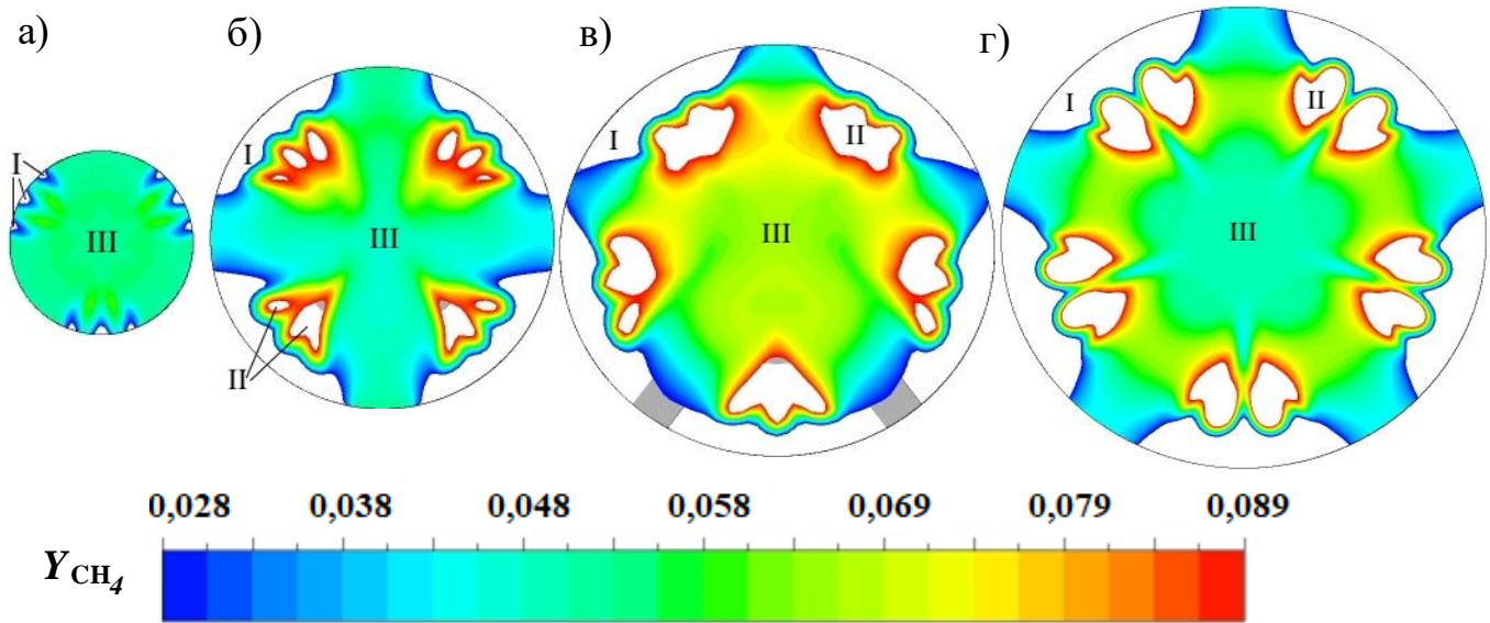
Рис. 14. Поля масової концентрації метану в поперечному перерізі x=0,275 м для циліндричних пальникових пристроїв з турбулізаторами потоку різної потужності: N_{п} = 30 кВт (а); N_{п} = 110 кВт (б); N_{п} = 155 кВт (в); N_{п} = 200 кВт (г); I, II – зони з надлишковим вмістом повітря і природного газу відповідно; III – зона утворення суміші в концентраційних межах займання.
