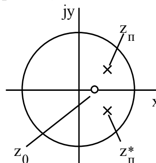
Рис. 3. Положення нуля і полюсів на z -площині
